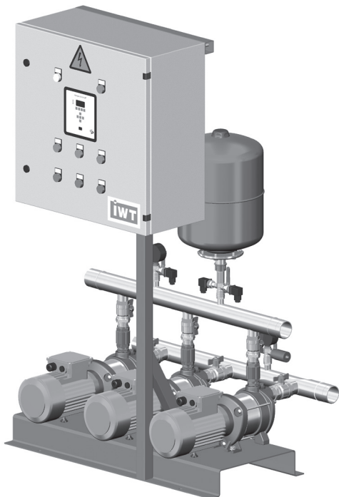
Насосна установка Hydro-Set DPHMC з частотними перетворювачами фірми ABF
