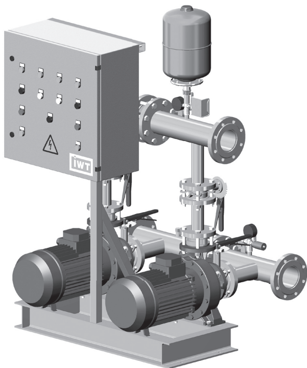
Насосна установка пожежогасіння Fire-Set 3D
