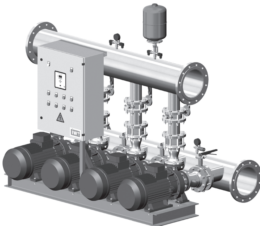
Насосна установка Hydro-Set 3D
