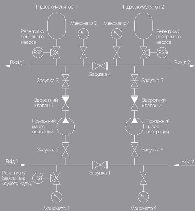
Гідравлічна схема Fire-Set DPV
