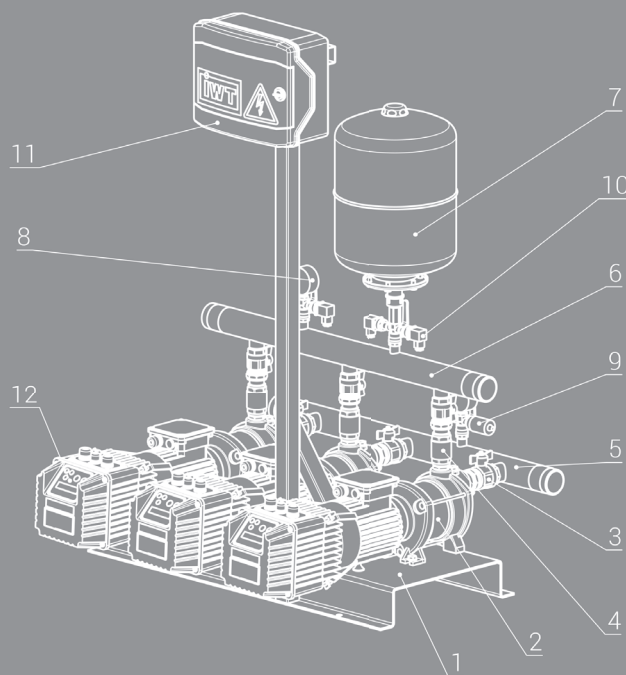
Насосна установка Hydro-Set DPHMC з частотними перетворювачами фірми Nastec
